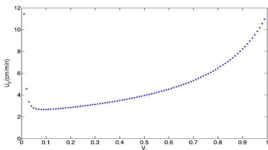
شکل (۶): تاثیر درصد حجمی الیاف در سرعت حرکت
